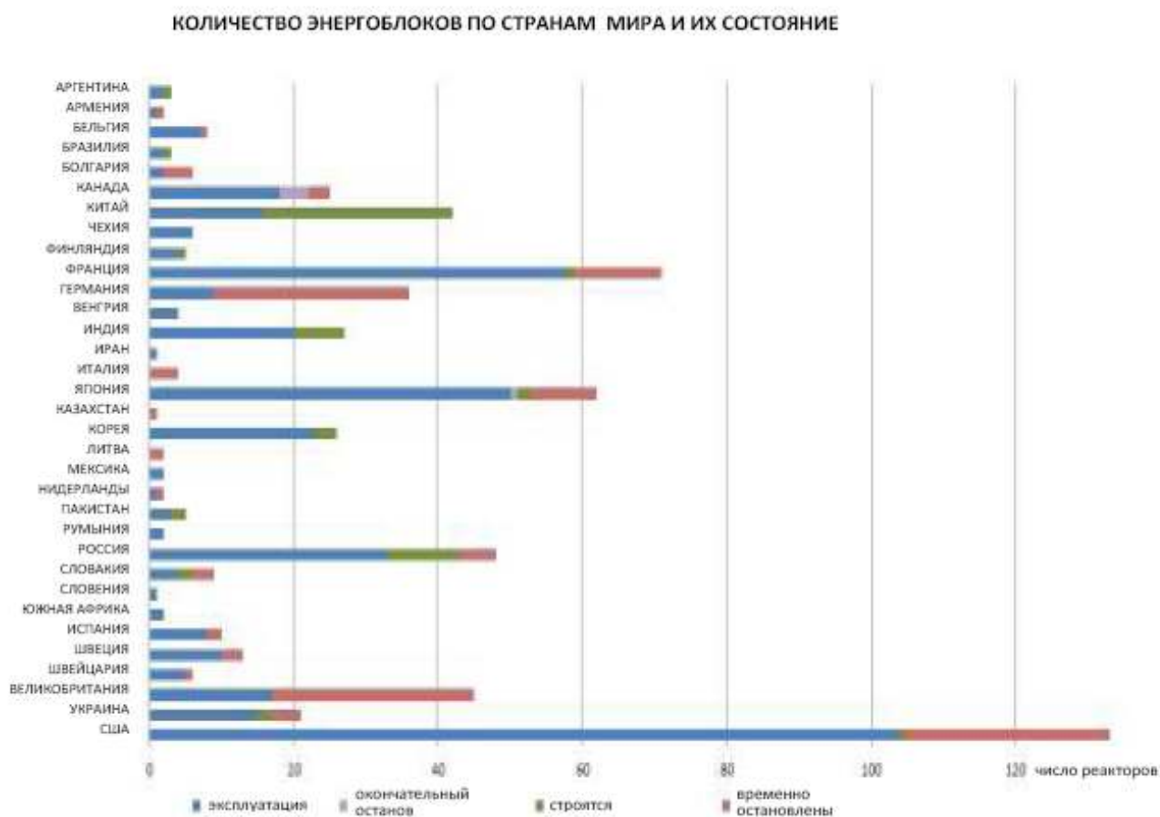
Рисунок 3 — Число ядерных энергоблоков по странам и их состояние.
