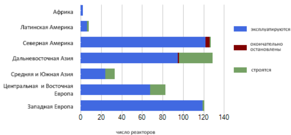
Рисунок 2 — распределение ядерных энергоблоков по регионам.
