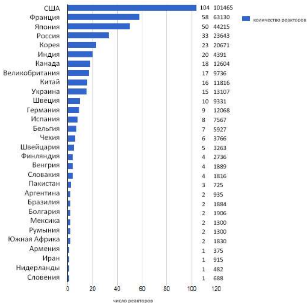
Рисунок 1 — Число ядерных энергоблоков, эксплуатируемых в странах мира.
